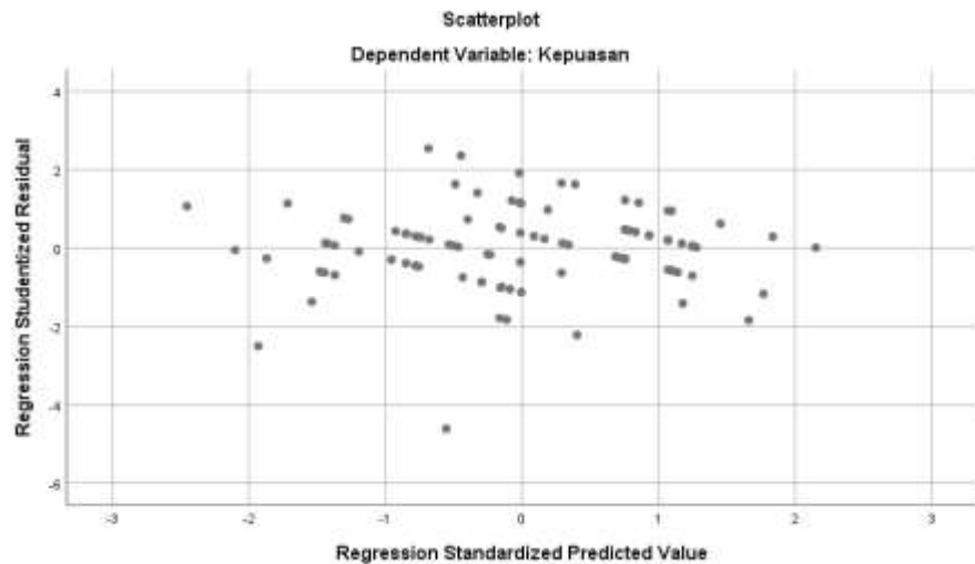
Gambar 3. Uji Heteroskedastisitas
