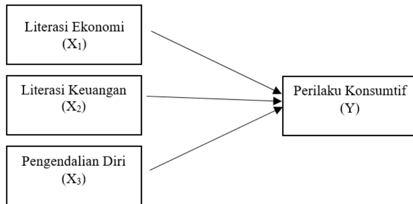
Gambar 1. Kerangka konseptual.
